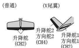
(3) 直升机的舵机连接方法示意图
